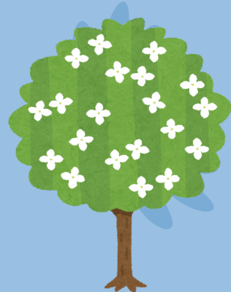
L'arbre Tree
