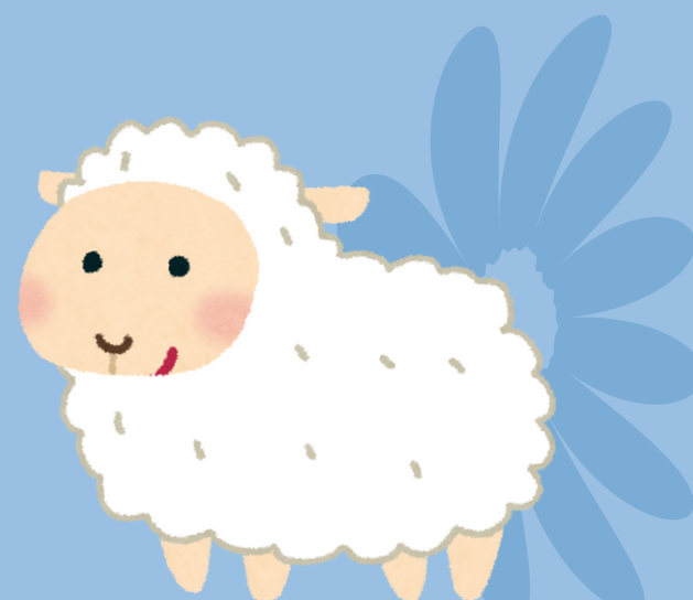
L'agneau Lamb
